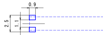
推奨パッド寸法 Recommended Pad Pattern
